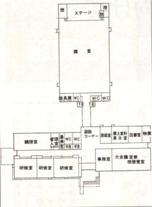
平面図
