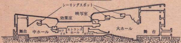
西側断面図
