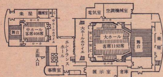
一階平面図
