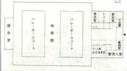
十二所体育館平面図
