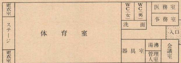
花岡体育館平面図
