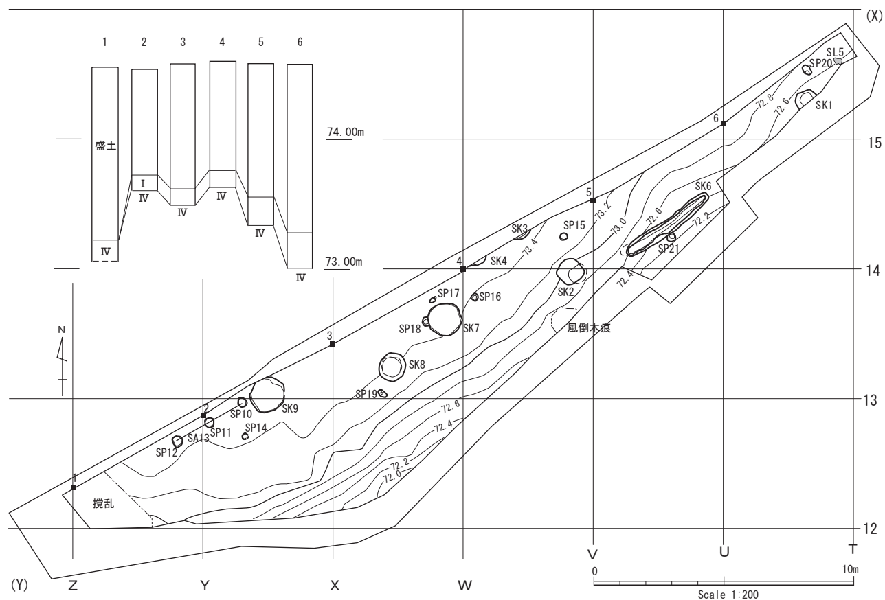
図3 遺構配置図
