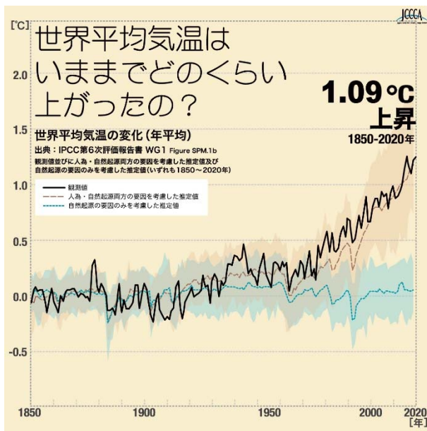
図1-2 世界平均気温の変化（1850～2020年・観測）
