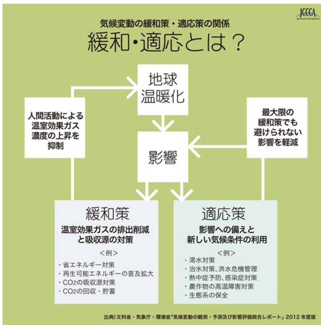
図 5-1 緩和策と適応策の関係
