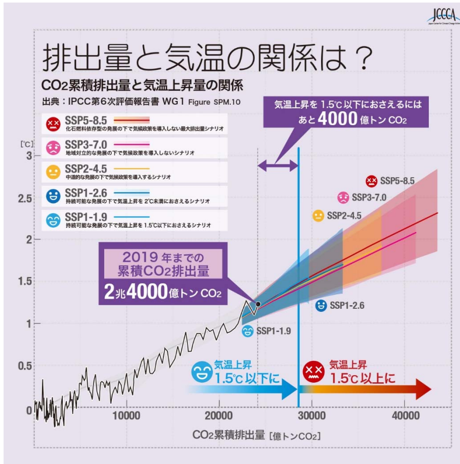
図 1-4 CO 2 累積排出量と気温上昇量の関係
