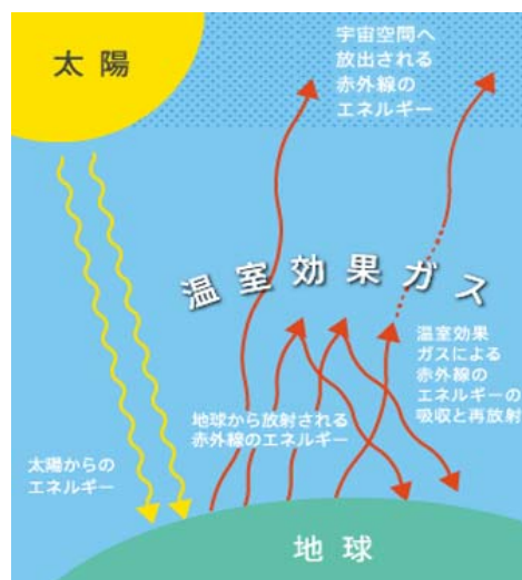
図 1-1 温室効果ガスによって気温が上がる仕組み
