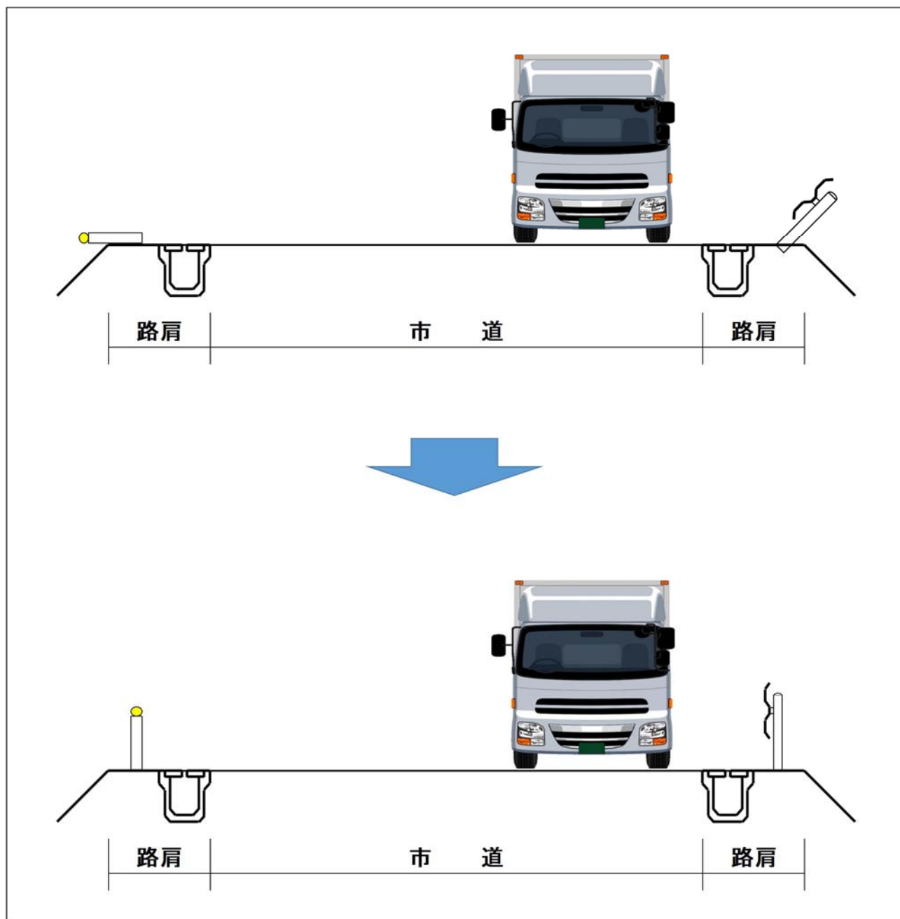
参考に想定される判断基準の図（道路附属物工の参考図）
