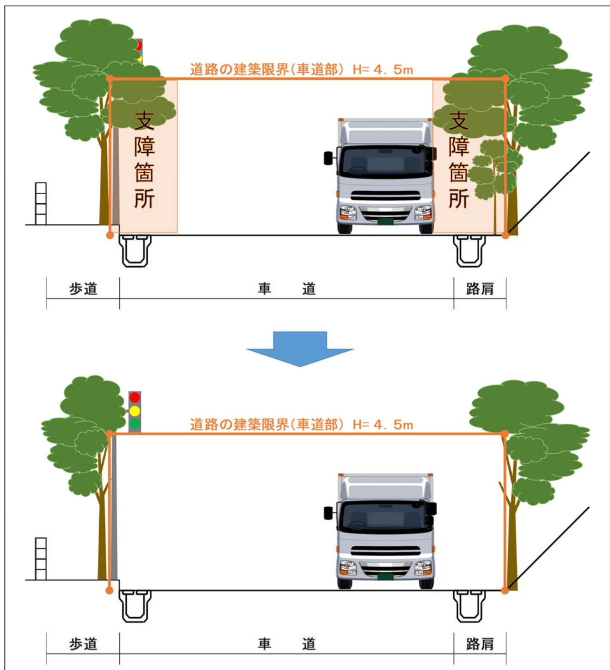
参考想定される判断基準の図（植栽維持工の参考図1） （ 車 道 部 ）
