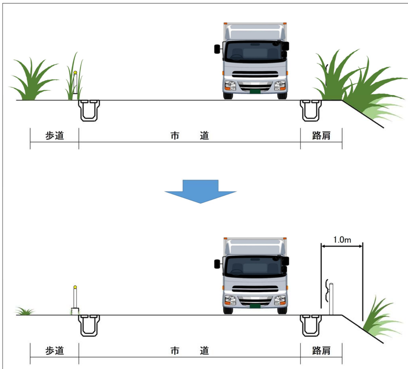
参考に想定される判断基準の図（除草工の参考図）
