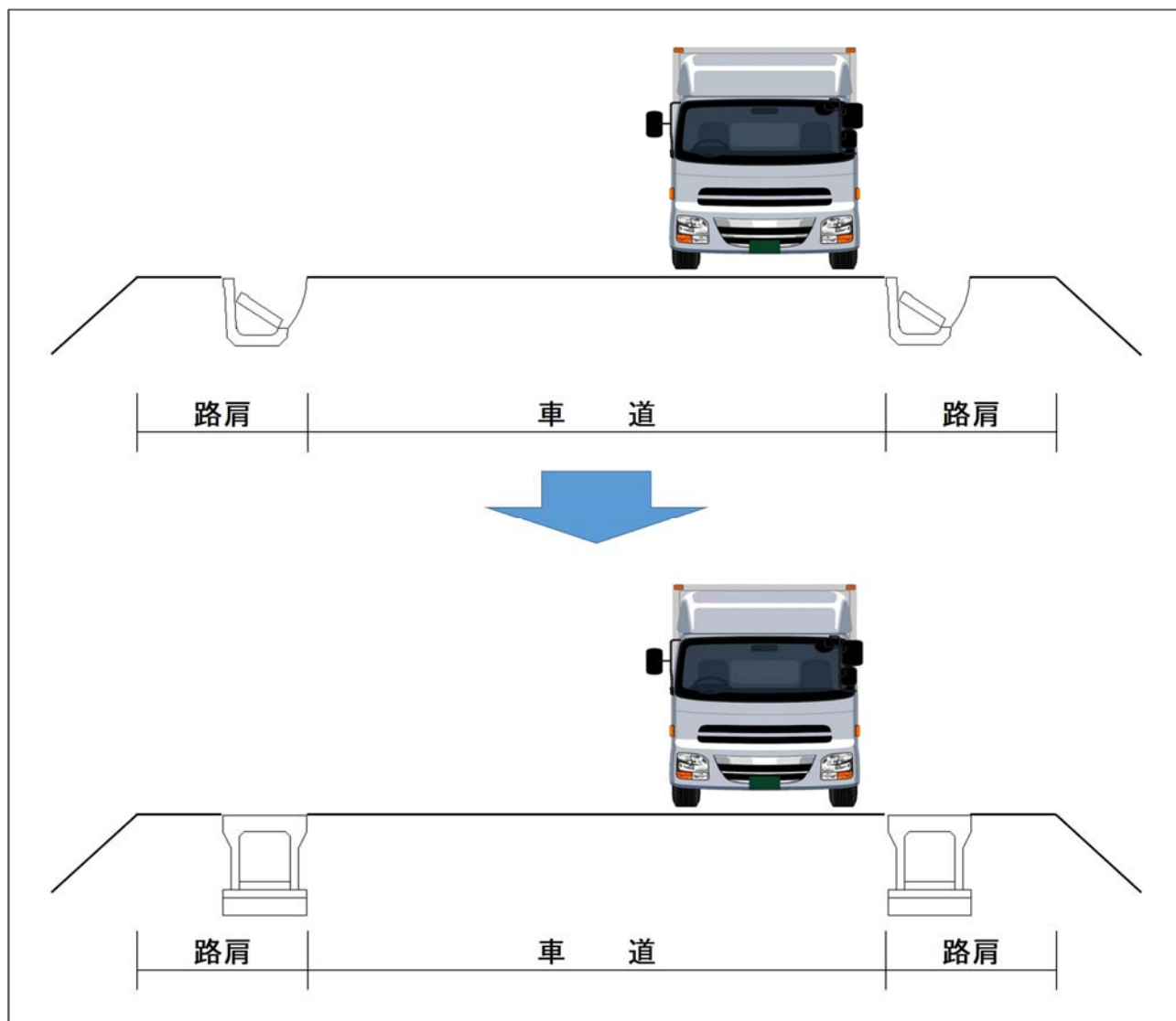
参考に想定される判断基準の図（排水構造物工の参考図）
